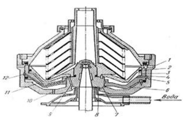
Рис. 36. Устройство барабана самоочищающегося сепаратора СЦС-3: 1 - разгрузочное отверстие; 2 - запирающий поршень; 3,6 - водяные полости; 4,7,9,10 - отверстия, 5 - сливной канал, 8 - камера; 11 - канал; 12 - кольцевой паз.
