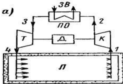
Рис. 37 Схема простейшей ВХУ.
