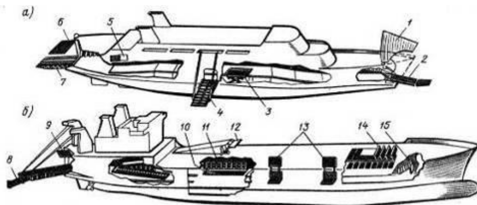
Рис. 34. Возможные схемы устройств для горизонтальной обработки судов: а) - на паромках; б) - на ролкерах; 1-обтекатель; 2 - носовая аппарель; 3-подъемник; 4-бортовая аппарель; 5-бортовой лацпорт; 6-закрытие комового проема; 7-кормовая аппарель; 8-угловая аппарель; 9-закрытие кормового проема; 10-пандус; 11-закрытие проема; 12-герметизированные закрытия пандусов; 13-лацпорты; 14-люки; 15-закрытие носового проема.
