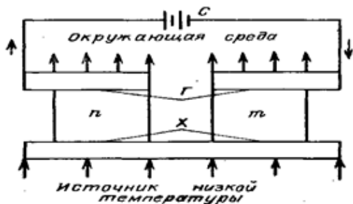
Рис.38 Схема термоэлемента
