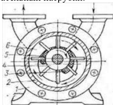
Рис. 6. Водокольцевой насос: 1-крышка; 2-корпус; 3-всасывающее отверстие; 4-ротор; 5-нагнетательное отверстие; 6 - водяное кольцо.
