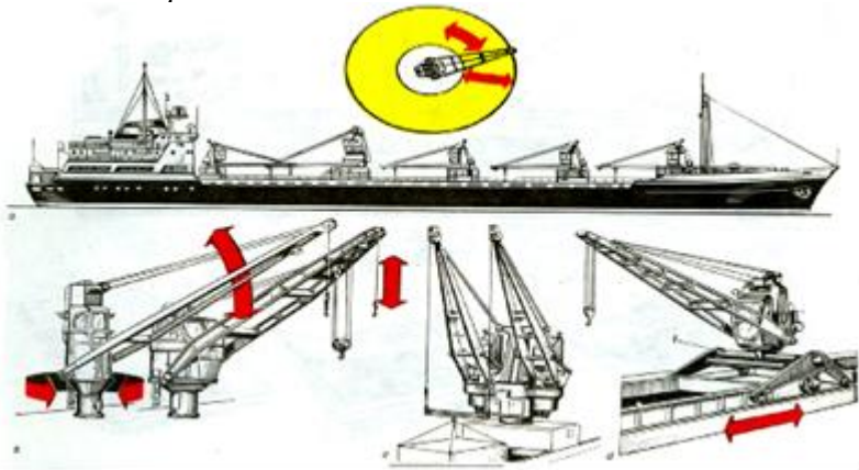
Рис. 32 Поворотные краны
