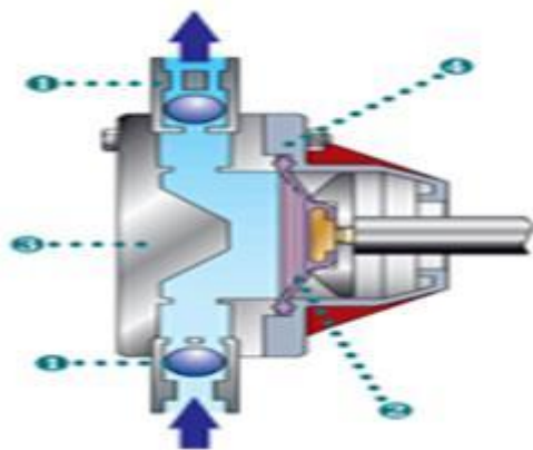
Рис. 15 Мембранный насос
