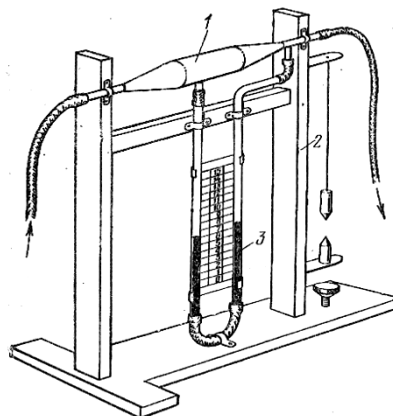
Рис. 2. Установа для перевірки рівняння Бернуллі
